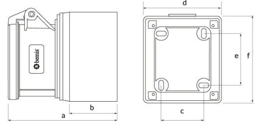
TEKNİK RESİM
