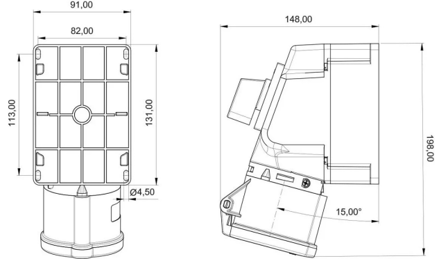
TEKNİK RESİM
