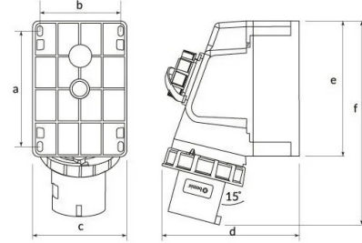
Ölçüler / Dimensions (mm)
