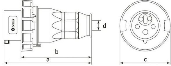
Ölçüler / Dimensions (mm)
