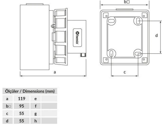
TEKNİK RESİM
