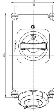
TEKNİK RESİM
