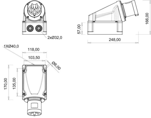
TEKNİK RESİM
