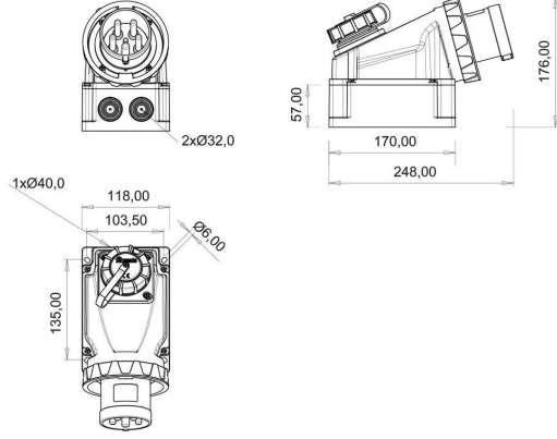
TEKNİK RESİM
