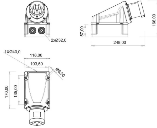
TEKNİK RESİM
