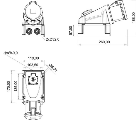
TEKNİK RESİM
