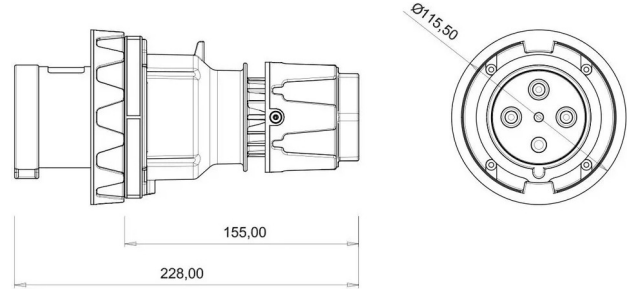
TEKNİK RESİM
