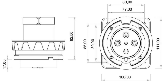
TEKNİK RESİM
