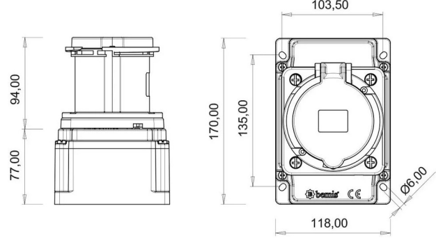
TEKNİK RESİM
