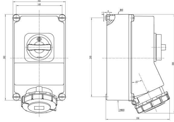
TEKNİK RESİM
