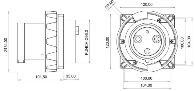
TEKNİK RESİM
