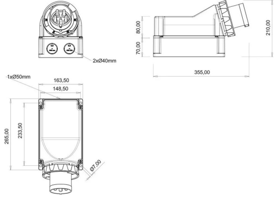
TEKNİK RESİM
