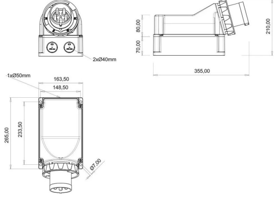
TEKNİK RESİM
