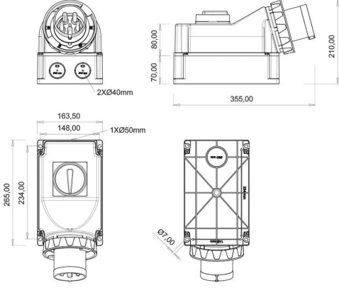
TEKNİK RESİM
