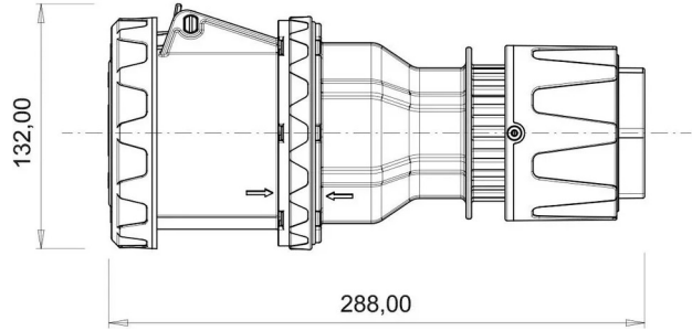
TEKNİK RESİM
