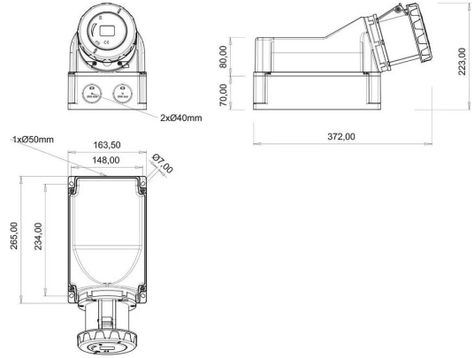
TEKNİK RESİM
