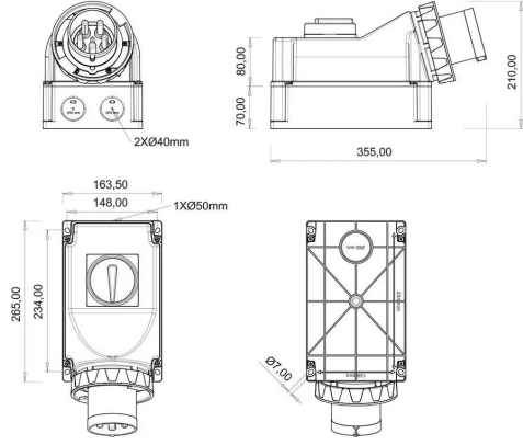
TEKNİK RESİM
