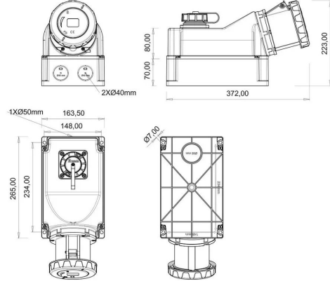
TEKNİK RESİM
