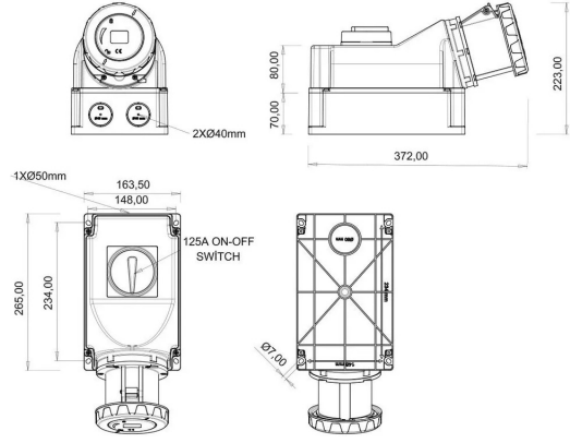
TEKNİK RESİM
