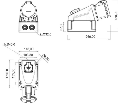
TEKNİK RESİM
