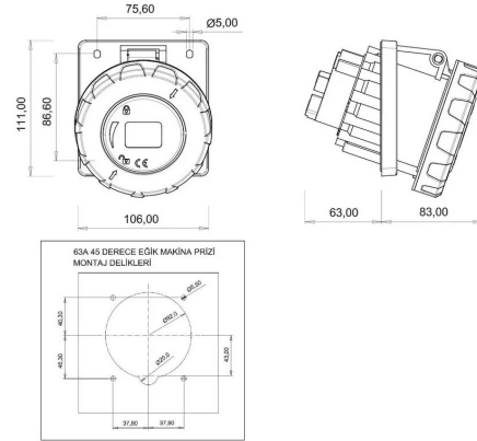
TEKNİK RESİM
