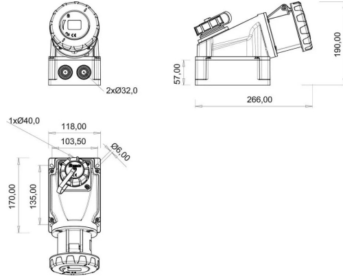
TEKNİK RESİM
