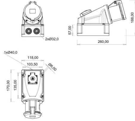
TEKNİK RESİM
