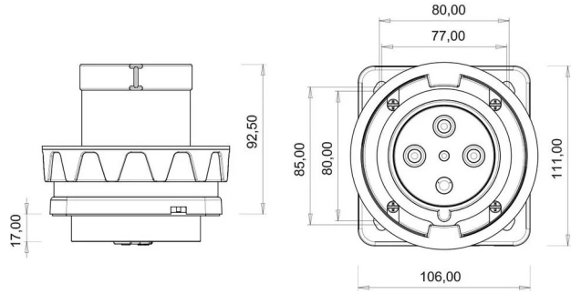
TEKNİK RESİM
