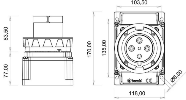
TEKNİK RESİM
