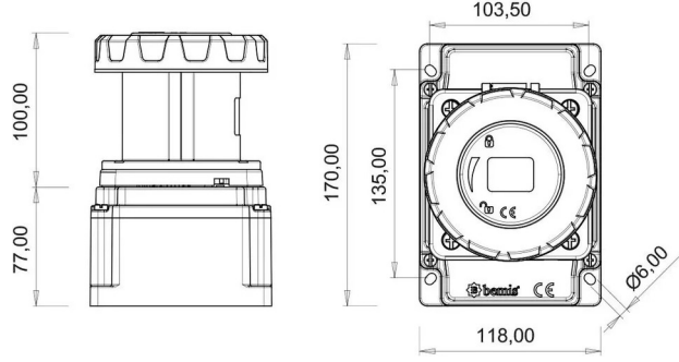
TEKNİK RESİM
