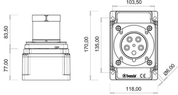
TEKNİK RESİM
