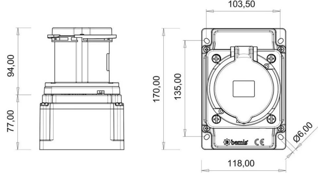
TEKNİK RESİM
