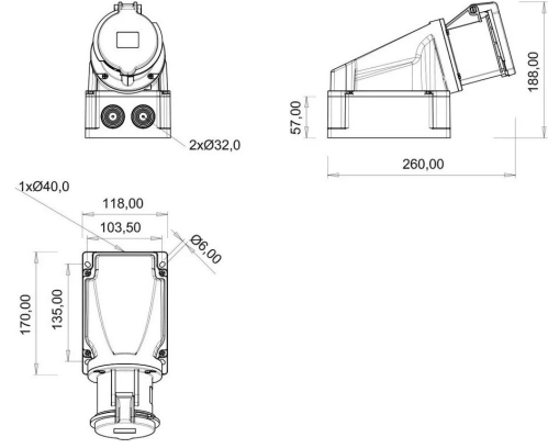
TEKNİK RESİM
