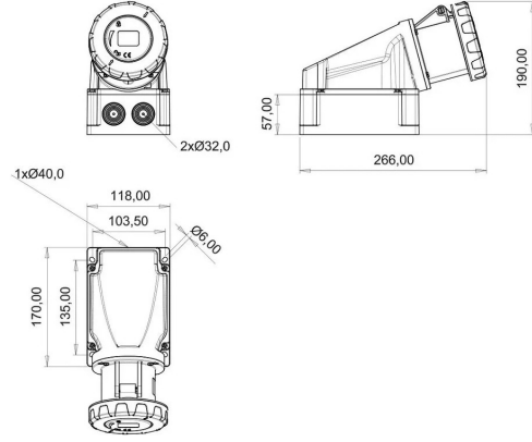
TEKNİK RESİM
