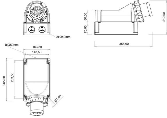
TEKNİK RESİM
