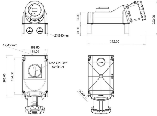
TEKNİK RESİM
