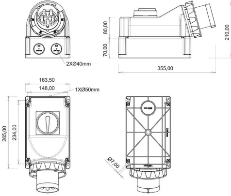
TEKNİK RESİM
