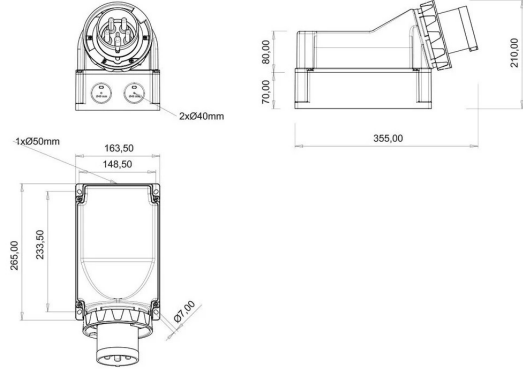
TEKNİK RESİM
