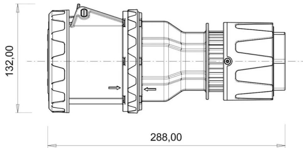
TEKNİK RESİM
