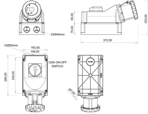
TEKNİK RESİM
