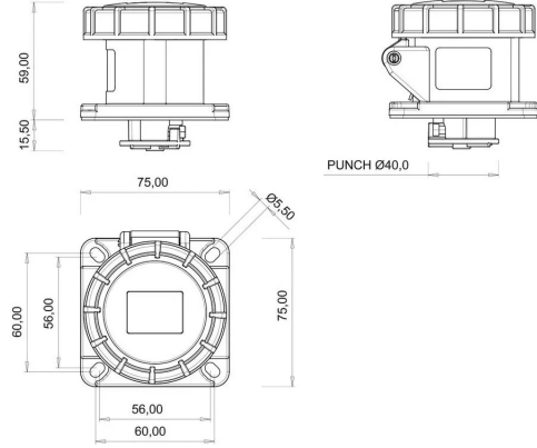
TEKNİK RESİM
