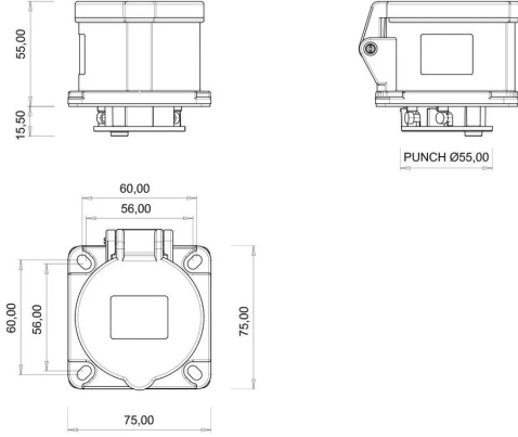
TEKNİK RESİM
