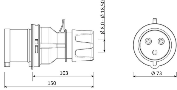
TEKNİK RESİM
