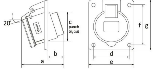
TEKNİK RESİM
