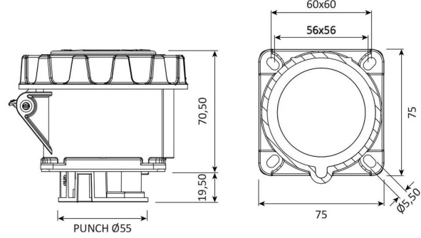
TEKNİK RESİM
