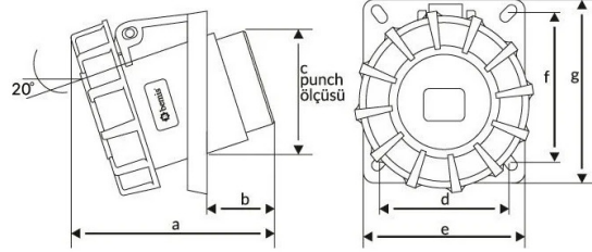
TEKNİK RESİM
