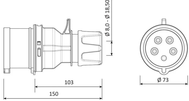
TEKNİK RESİM
