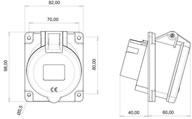
TEKNİK RESİM
