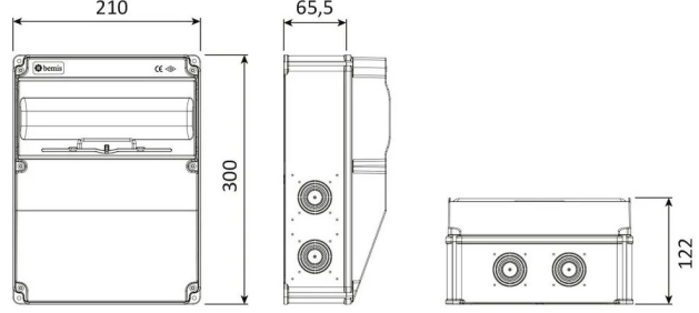
TEKNİK RESİM
