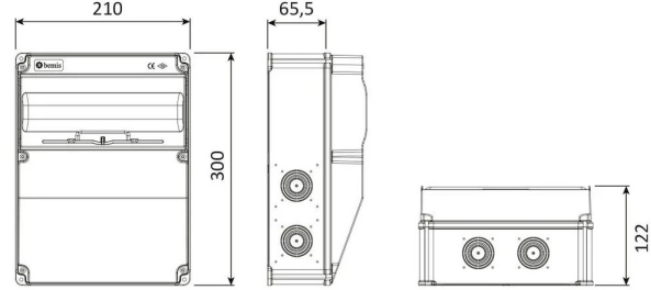
TEKNİK RESİM
